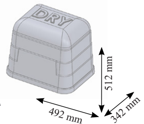
KOMPRESOROVÁ JEDNOTKA
